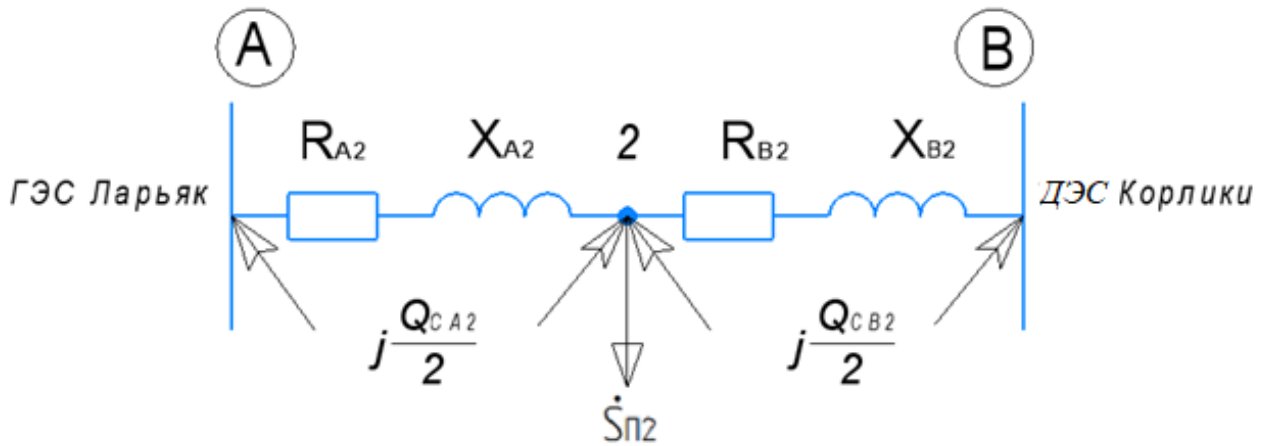
Рисунок 3.6 – Схема замещения участка электрической сети ЛДП 2
