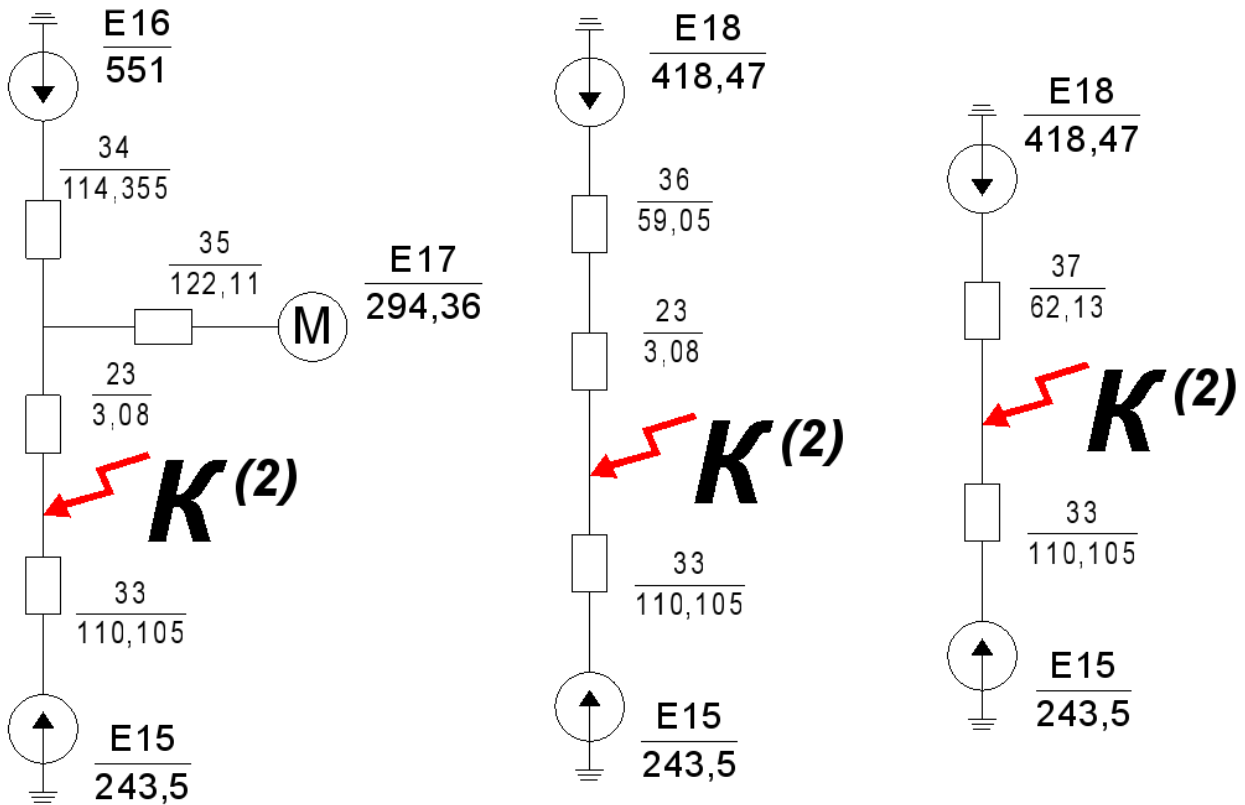
Рисунок 8.6 – Завершение преобразования схемы замещения ЭЭС прямой последовательности в именованных единицах
