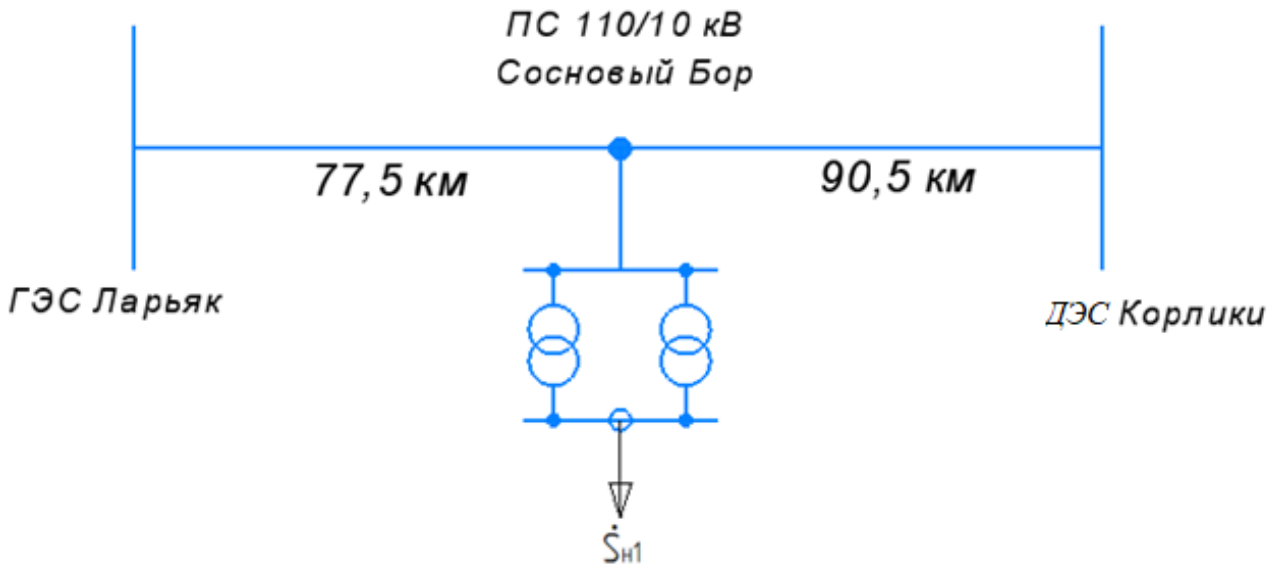
Рисунок 3.1 – Схема участка электрической сети ЛДП 1
