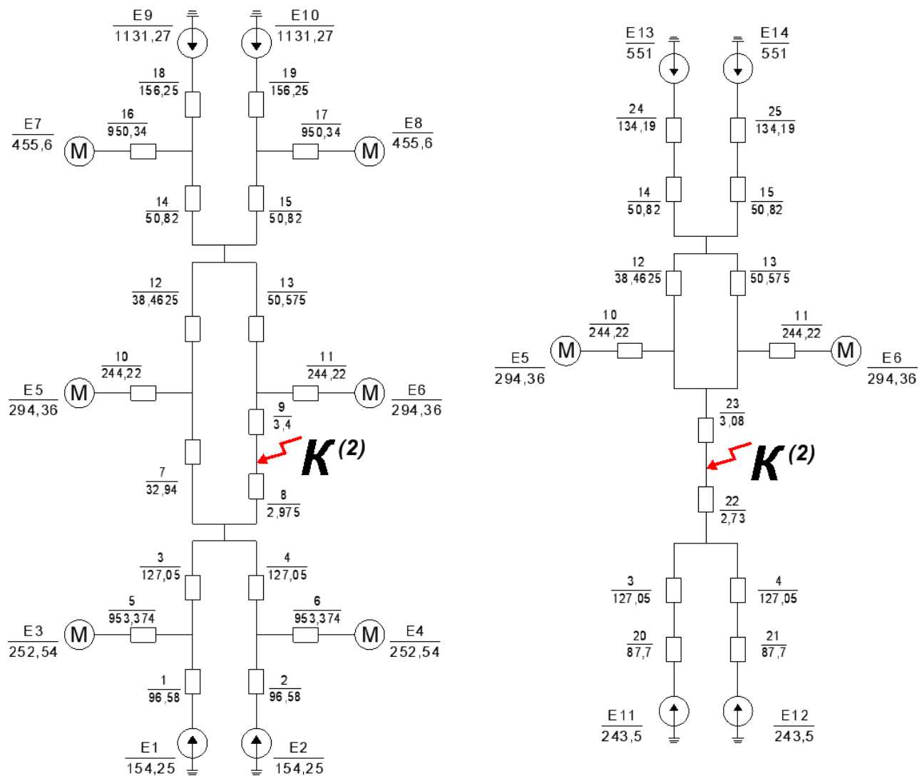
Рисунок 8.1 – Преобразование схемы замещения ЭЭС прямой последовательности в именованных единицах
