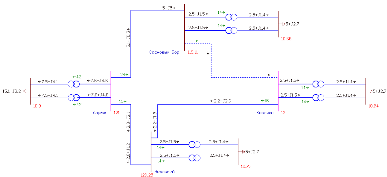
Рисунок 3.11 – Схема электрической сети в послеаварийном режиме при отключении линии Сосновый Бор - Корлики
