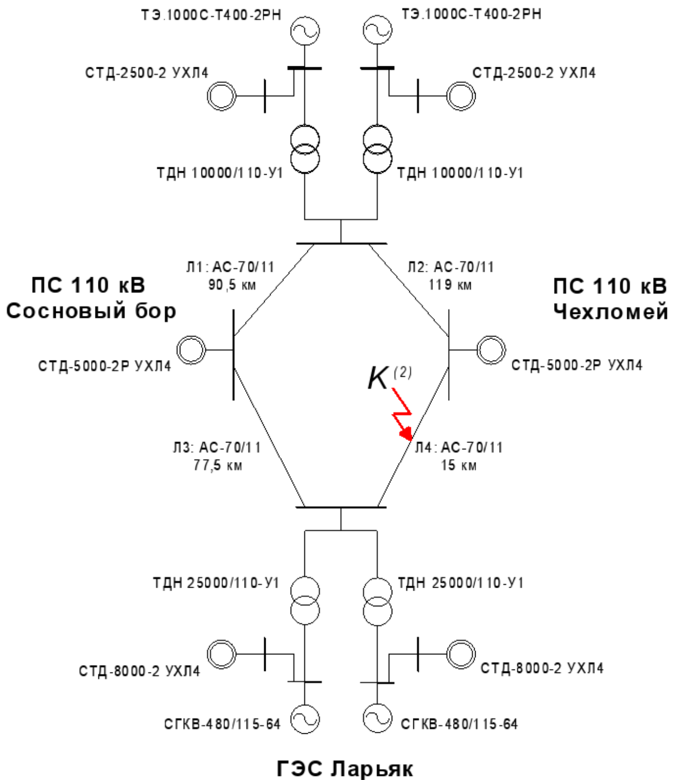
Рисунок 7 – Принципиальная схема ЭЭС для расчёта переходных процессов
