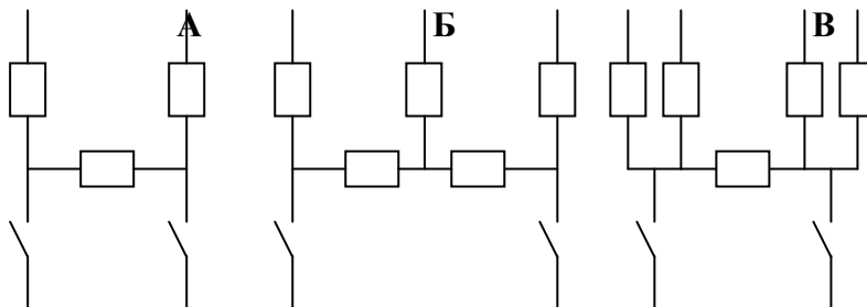
Рисунок 2.6 – Схемы РУ-35/110 кВ
