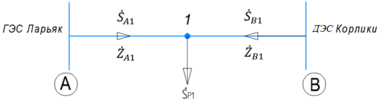
Рисунок 3.3 – Топологическая схема участка электрической сети ЛДП 1
