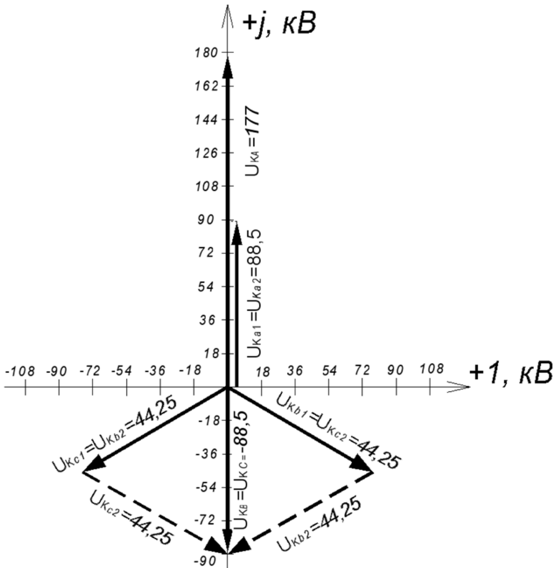
Рисунок 9.4 – Векторная диаграмма напряжений в месте двухфазного КЗ
