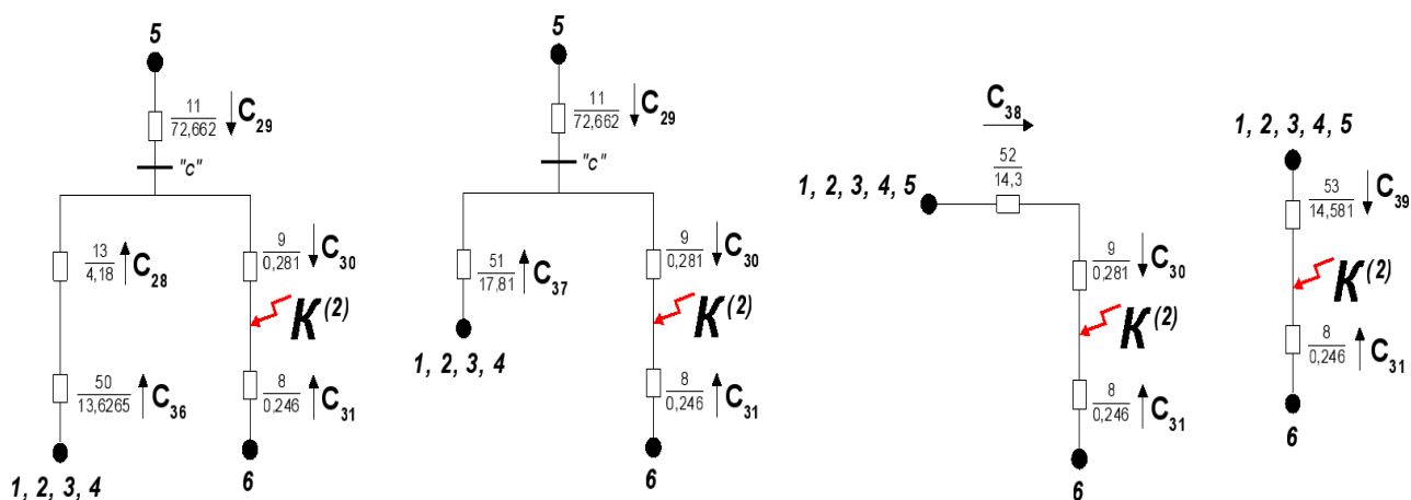
Рисунок 8.12 – Завершение преобразования части схемы ЭЭС прямой последовательности с узлами с, d и e
