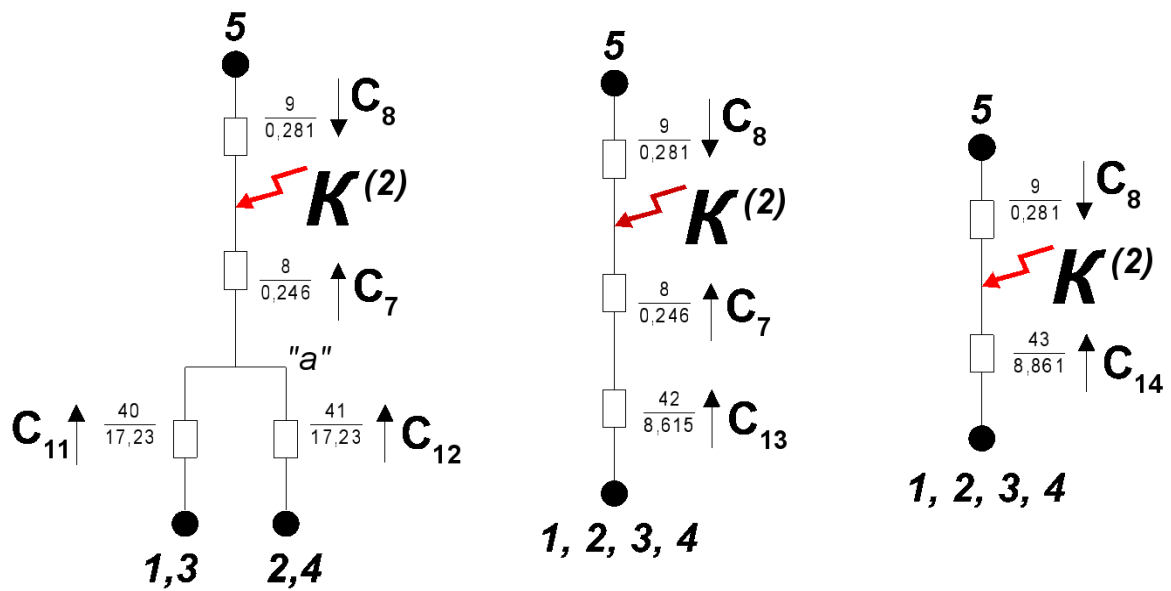
Рисунок 8.8 – Завершение преобразования части схемы ЭЭС прямой последовательности с узлами a и b
