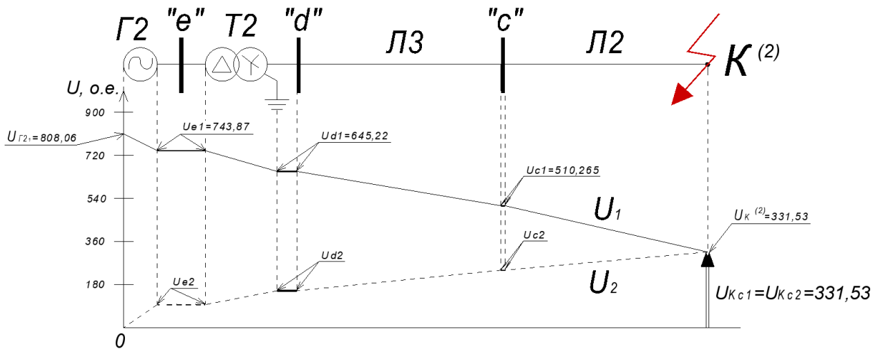
Рисунок 10.2 – Эпюра симметричных составляющих напряжений для части схемы ЭСС с узлами с, d и e
