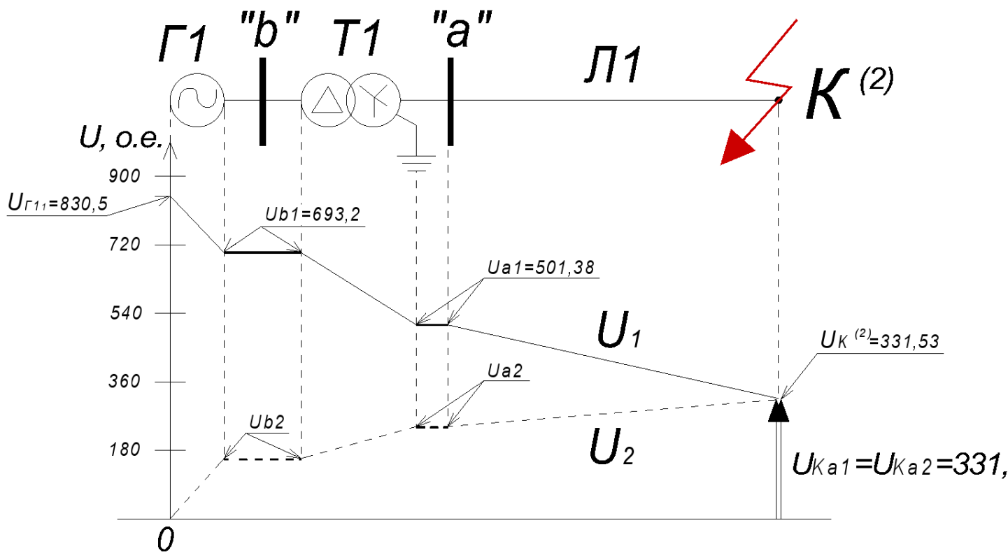
Рисунок 10.1 – Эпюра симметричных составляющих напряжений для части схемы ЭСС с узлами a и b
