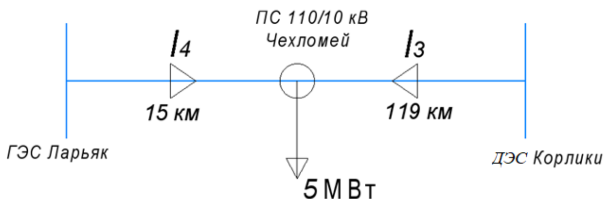
Рисунок 2.3 Схема линейного диспетчерского пункта 2
