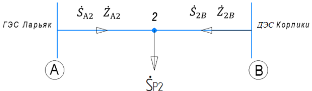
Рисунок 3.7 – Топологическая схема участка электрической сети ЛДП 2
