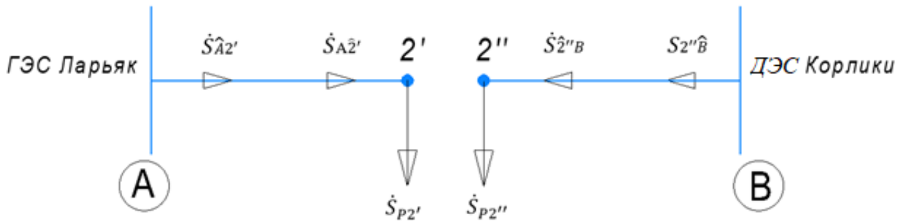
Рисунок 3.8 – Схема участка электрической сети ЛДП 2 с указанием точки потокораздела
