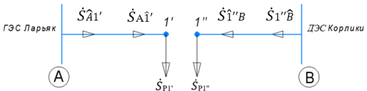
Рисунок 3.4 – Схема участка электрической сети ЛДП 1 с указанием точки потокораздела
