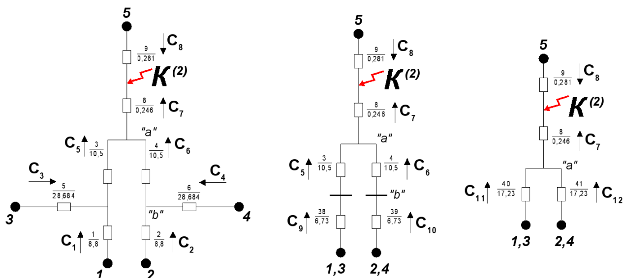
Рисунок 8.7 – Преобразование части схемы ЭЭС прямой последовательности с узлами a и b
