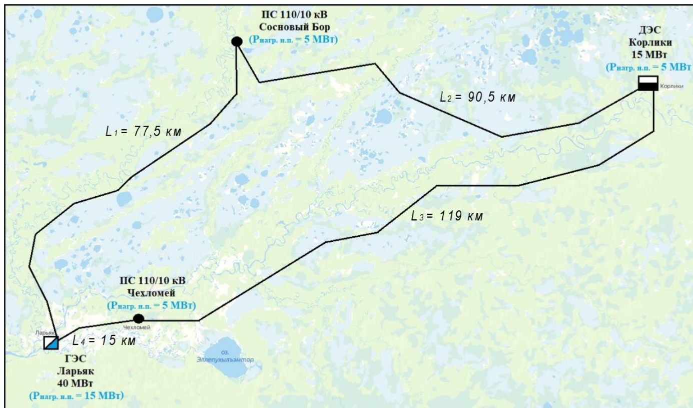
Рисунок 2.1 Схема электрической сети
