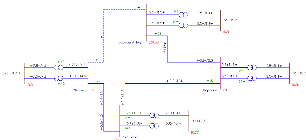
Рисунок 3.10 – Схема электрической сети в послеаварийном режиме при отключении линии Ларьяк – Сосновый Бор
