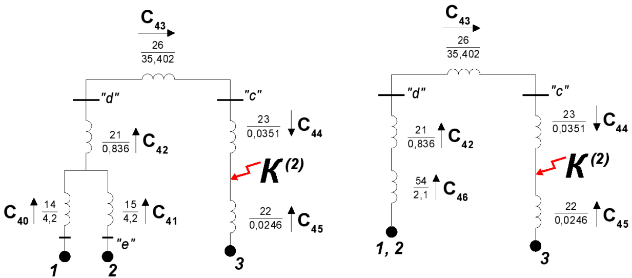
Рисунок 8.13 – Преобразование части схемы ЭЭС нулевой последовательности с узлами c , d и e
