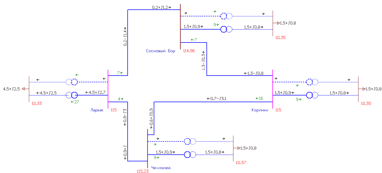
Рисунок 3.9 – Схема электрической сети в нормальном минимальном режиме
