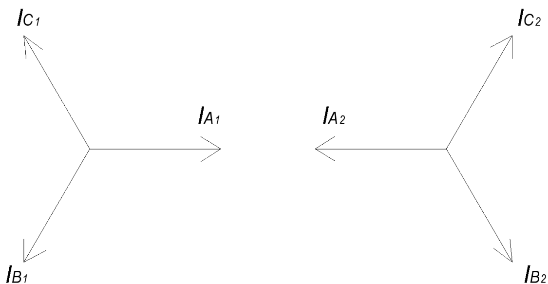
Рисунок 9.1 – Сориентированные вектора токов прямой и обратной последовательностей при двухфазном КЗ
