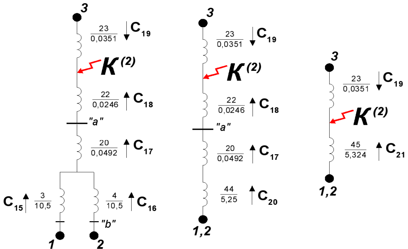
Рисунок 8.9 – Преобразование части схемы ЭЭС нулевой последовательности с узлами a и b
