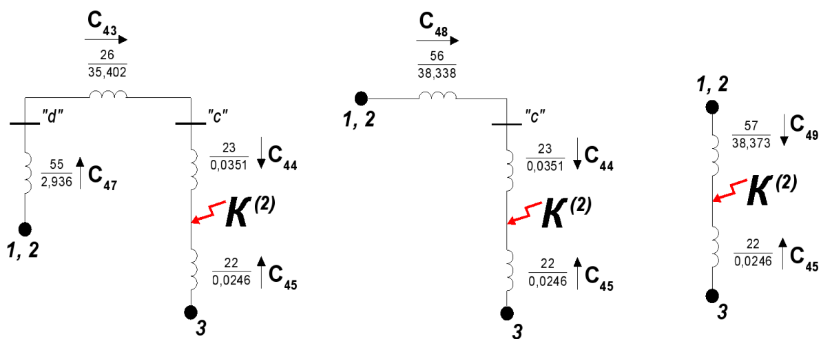
Рисунок 8.15 - Завершение преобразования части схемы ЭЭС нулевой последовательности с узлами c, d и e
