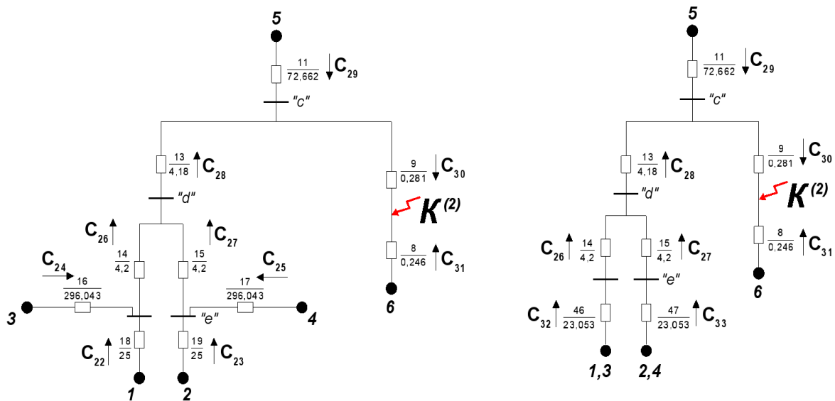
Рисунок 8.10 – Преобразование части схемы ЭЭС прямой последовательности с узлами c , d и e
