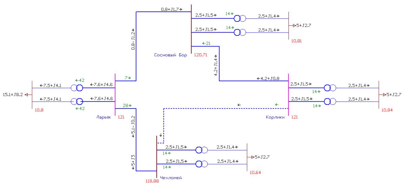
Рисунок 3.12 – Схема электрической сети в послеаварийном режиме при отключении линии Корлики - Чехломей
