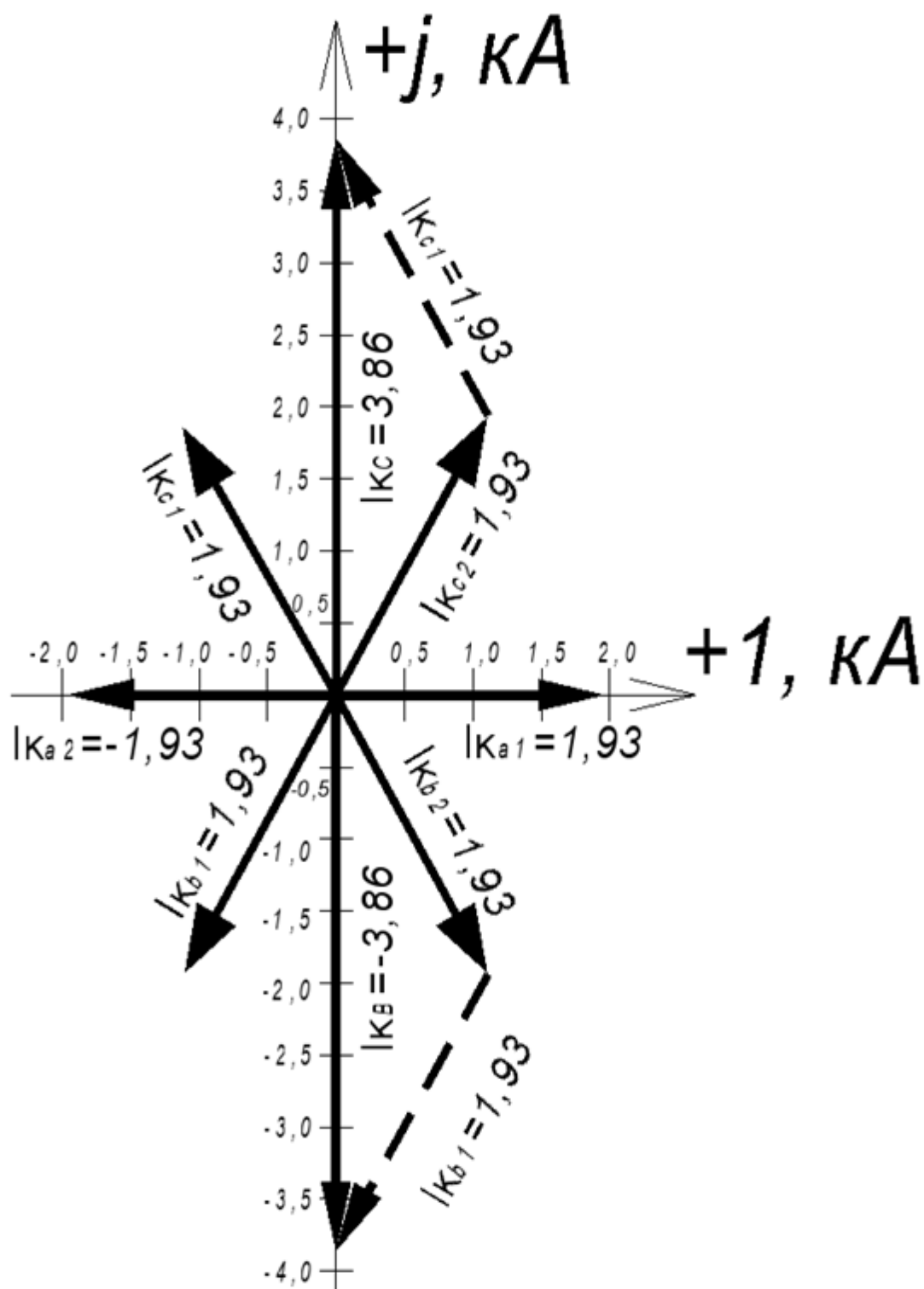
Рисунок 9.3 – Векторная диаграмма токов в месте двухфазного КЗ
