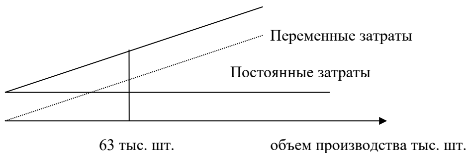
Рис.1. График безубыточности
